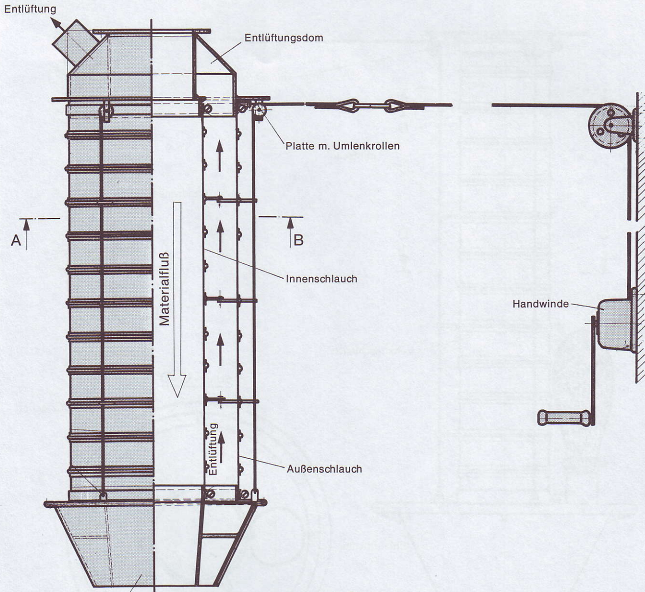
Schnitt A-B
