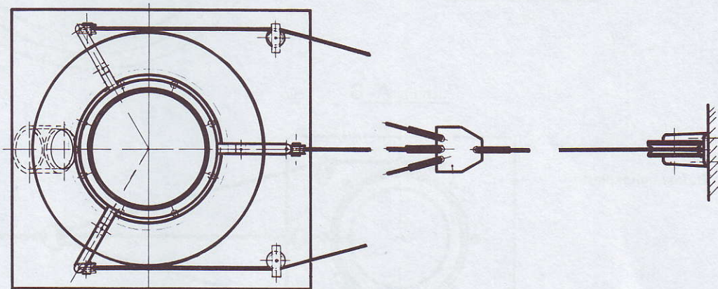
Schnitt A-B
